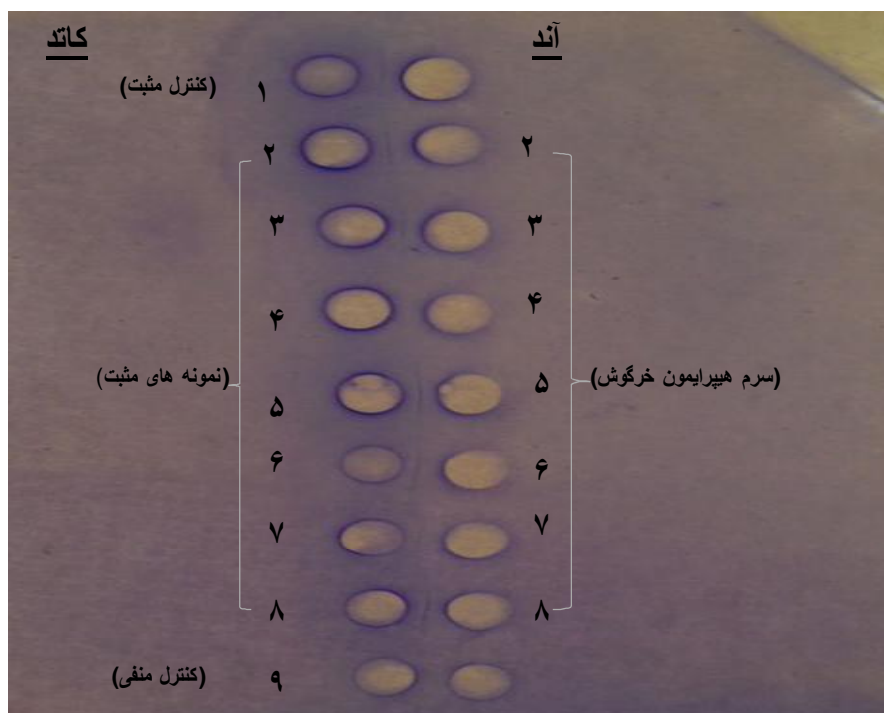
تصویر 3-1: روش کانترایمنوالکتروفورز روی اسلاید ژل آگاروز 1 درصد جهت تشخیص آنتی ژن های گردشی فاسیولا ژیگانتیکا در سرم گاو
