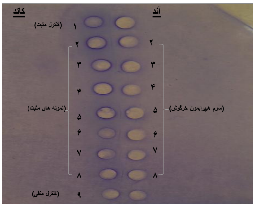
تصویر 4-1: نتایج آزمایش کانترایمنوالکتروفورز 8 نمونه سرم گاوان آلوده و غیر آلوده به فاسیولا ژیگانتیکا
